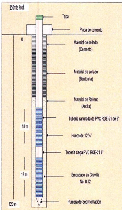
Figura 10. Pre-diseño del pozo a 150mts.
